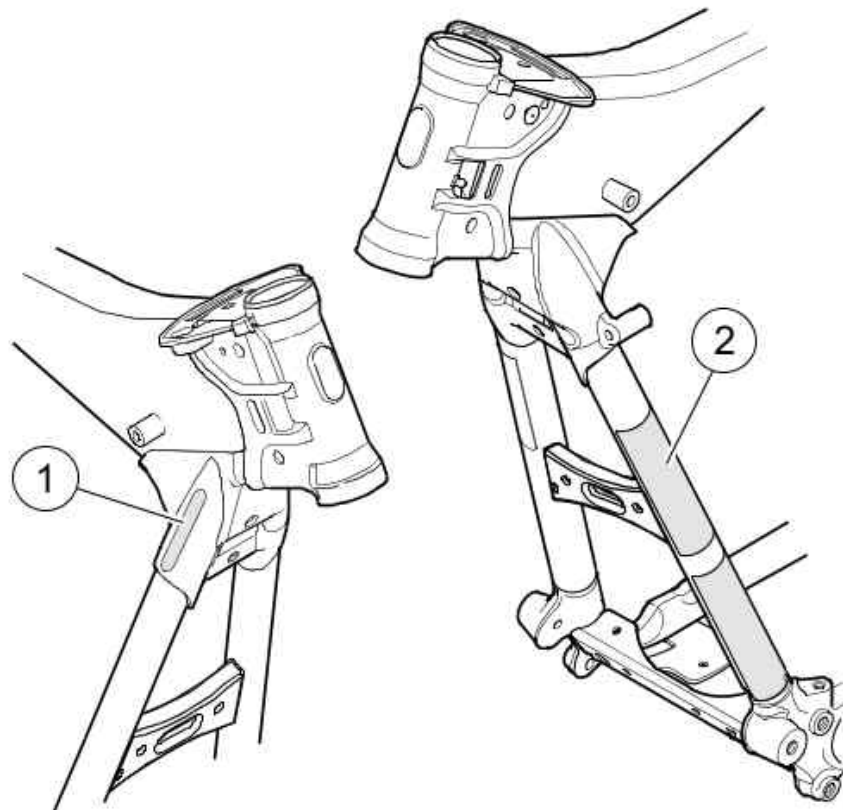
VIN Locations
